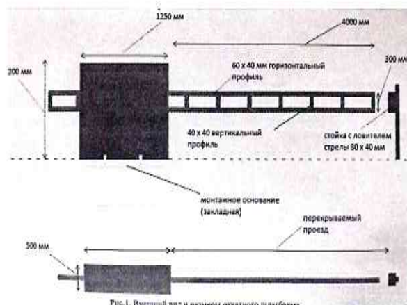
Рис. 1. Внешний вид и размеры откатного шлагбаума.
